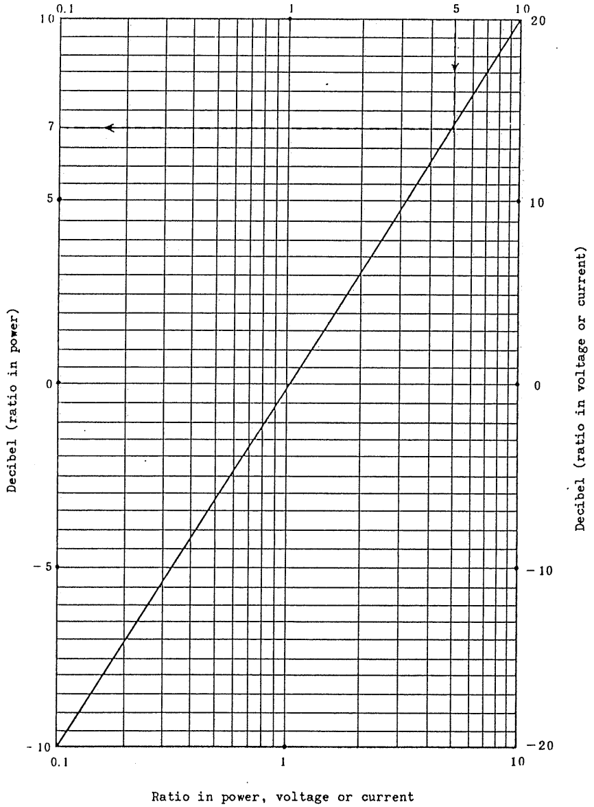
Decibel conversion chart
